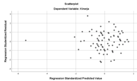
Gambar 1. Grafik Scatterplot
